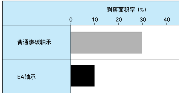
图7 耐剥落强度试验结果
