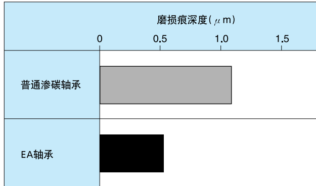
图8 通过试验机得到的磨损试验结果
