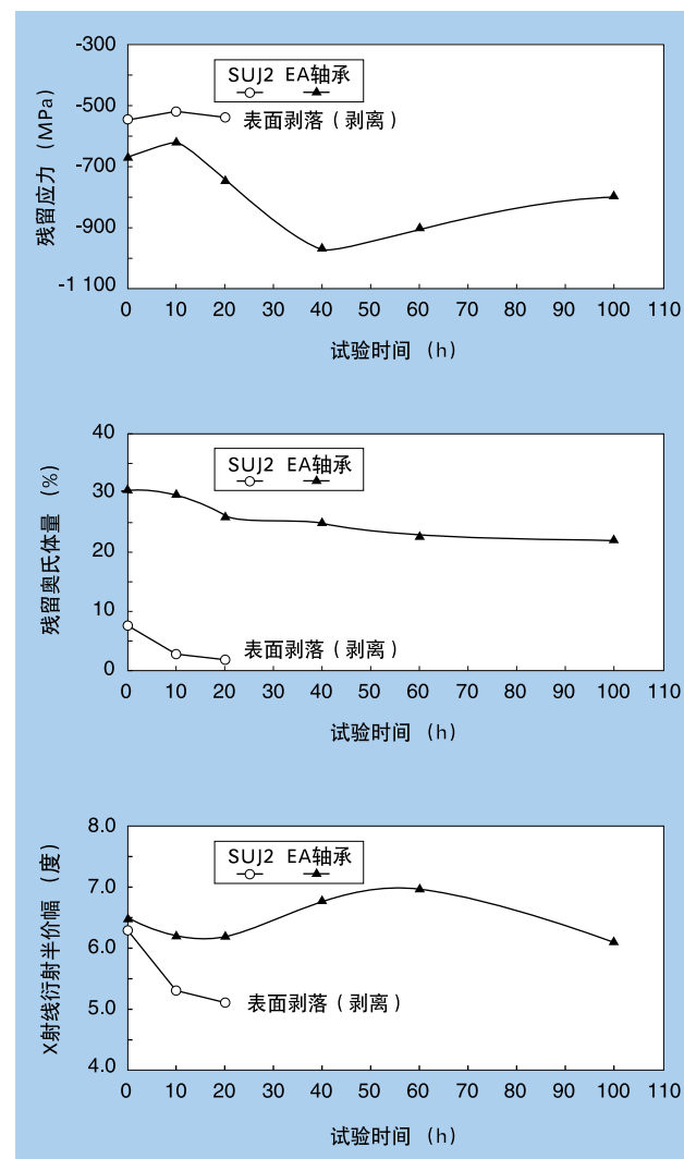
图3 异物侵入的滚动疲劳过程中轴承表面的材质变化
