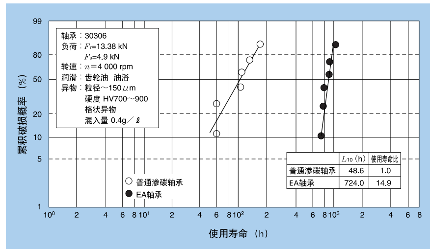
图5 异物侵入润滑条件下的使用寿命试验结果（2）
