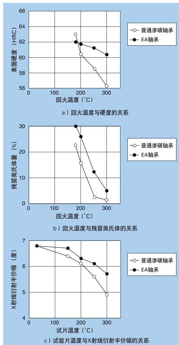
图2 标准渗碳轴承与EA轴承材质稳定性的比较
