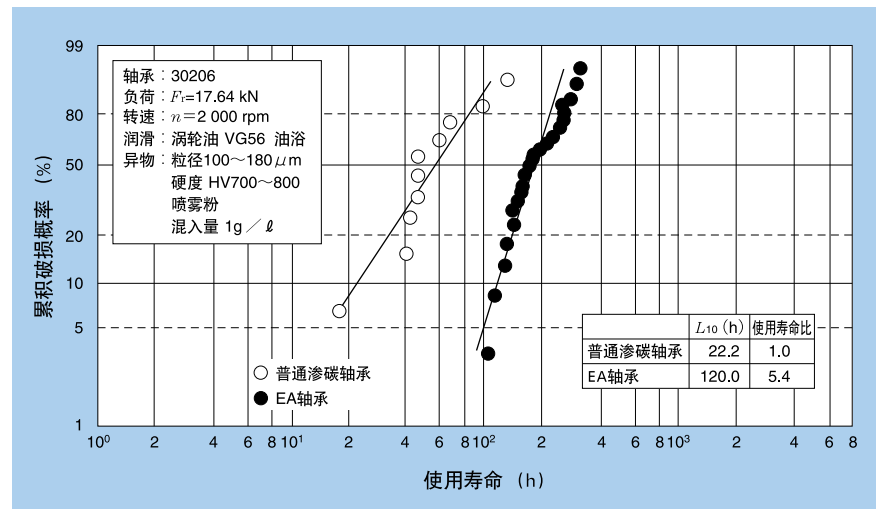
图4 异物侵入润滑条件下的使用寿命试验结果（1）
