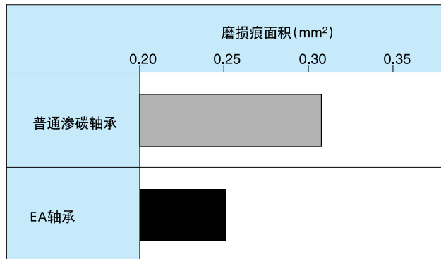
图9 磨蚀磨损试验结果
