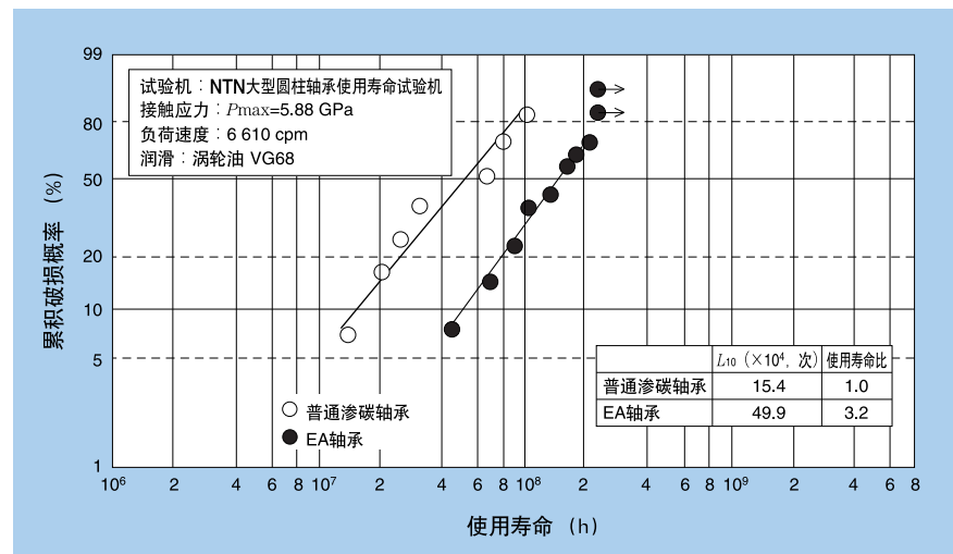
图6 清洁油润滑条件下的使用寿命试验结果
